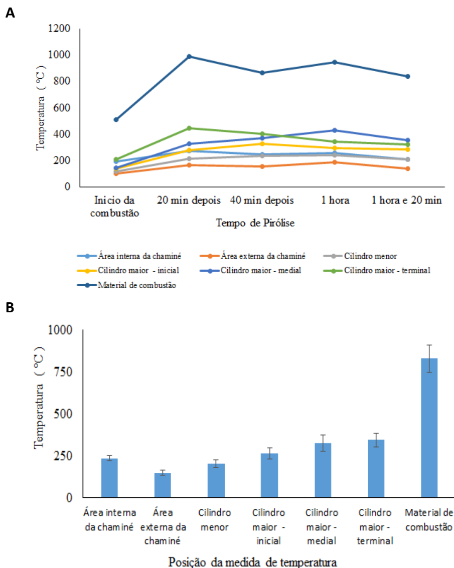
Figura 13. Análise da distribuição de temperatura a cada 20 minutos no forno de pirólise (A) e média da temperatura durante o processo (B)
